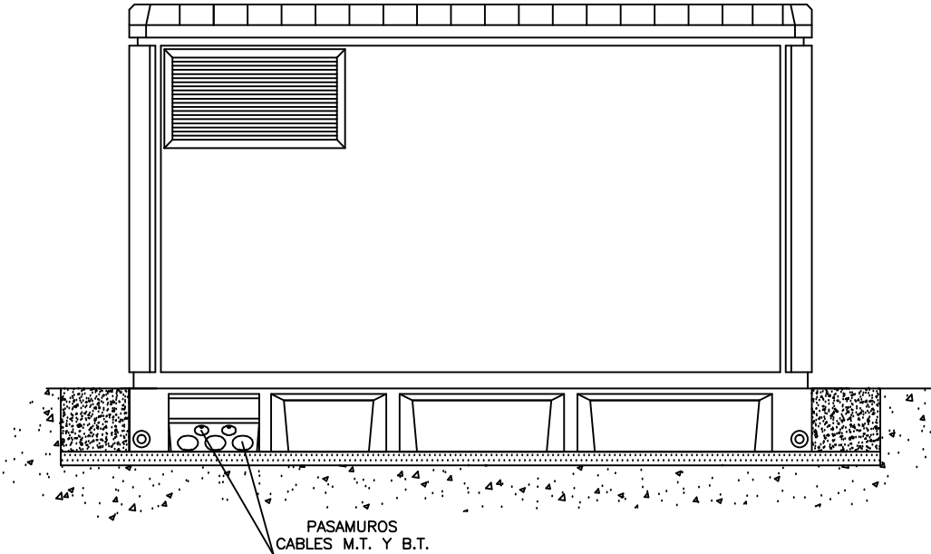
ALZADO POSTERIOR
