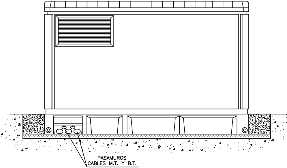
ALZADO POSTERIOR
