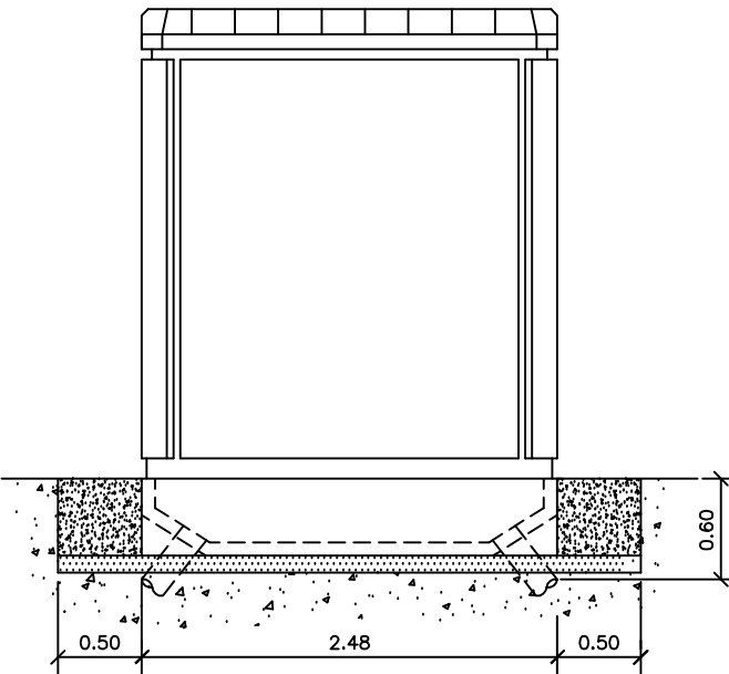
ALZADO LATERAL
